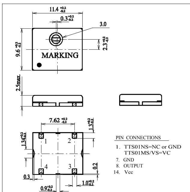
■外観寸法図
